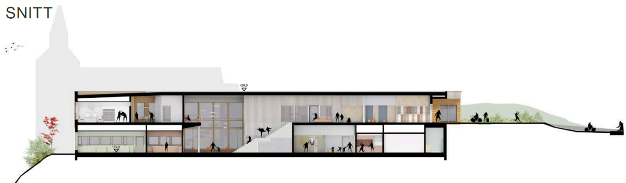
Snitt B 1:200
